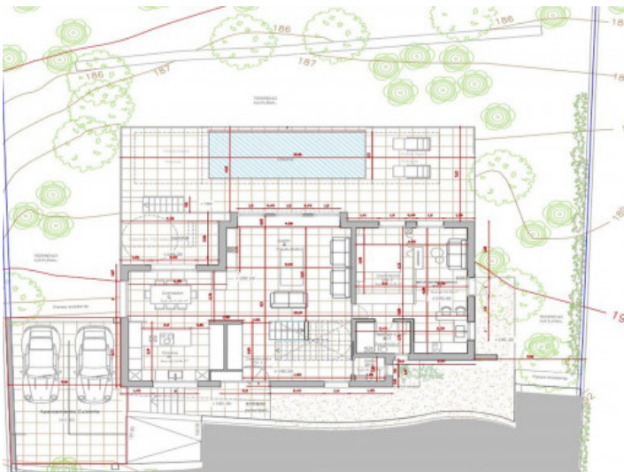
Grundriss Bauprojekt
