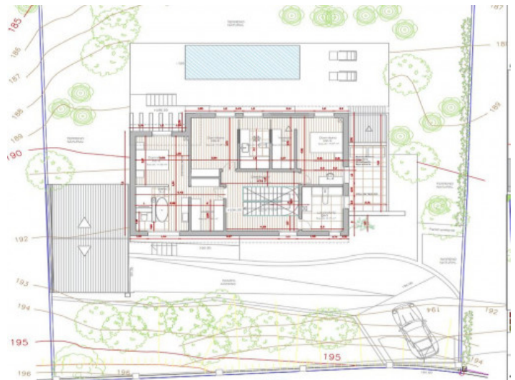
Grundriss Bauprojekt
