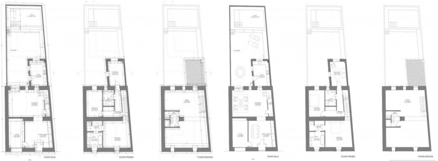
Grundriss
