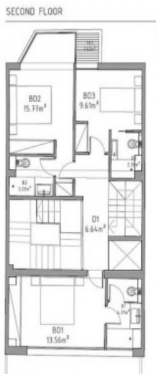
Bauzeichnung des oberen Stockwerkes
