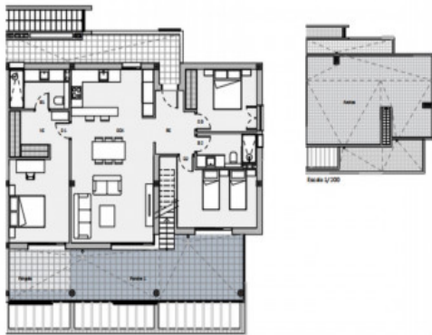
Grundriss
